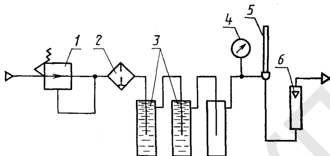
1—регулятор давления; 2—фильтр окончательной очистки; 3—поглощательные приборы; 4—манометр образцовый; 5—термометр; 6—ротаметр типа РМ
