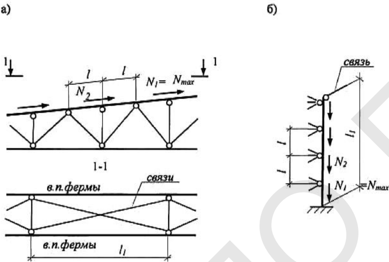
а) - пояса фермы; б) - ветви колонны
