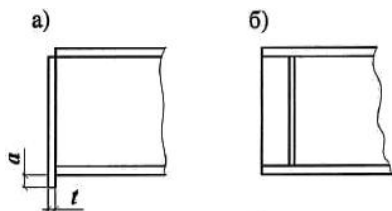
Рисунок 11 - Схема опорного ребра жесткости
