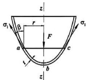
Рисунок 16 - Схема оболочки вращения
