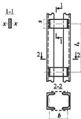
Рисунок 4 - Сквозной стержень с планками
